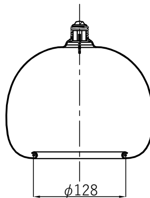
断面 A-A
