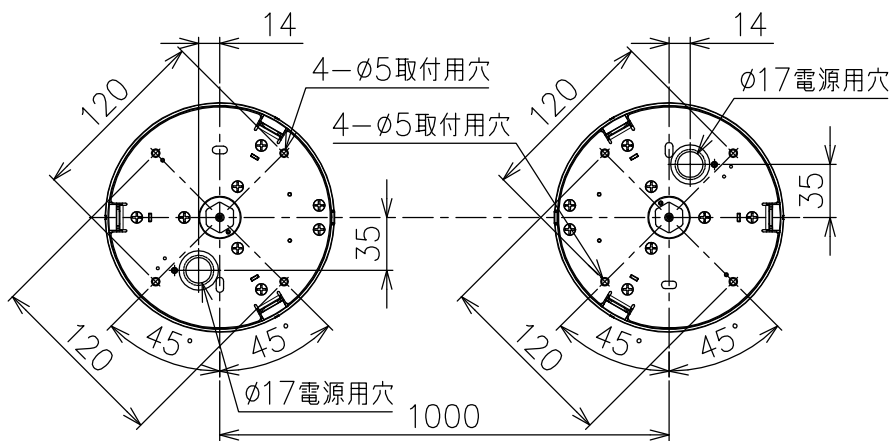
取付板詳細 S:1/5
