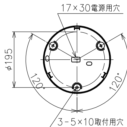
取付板詳細
